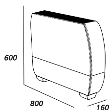
БлД/БпД(диз.1)
